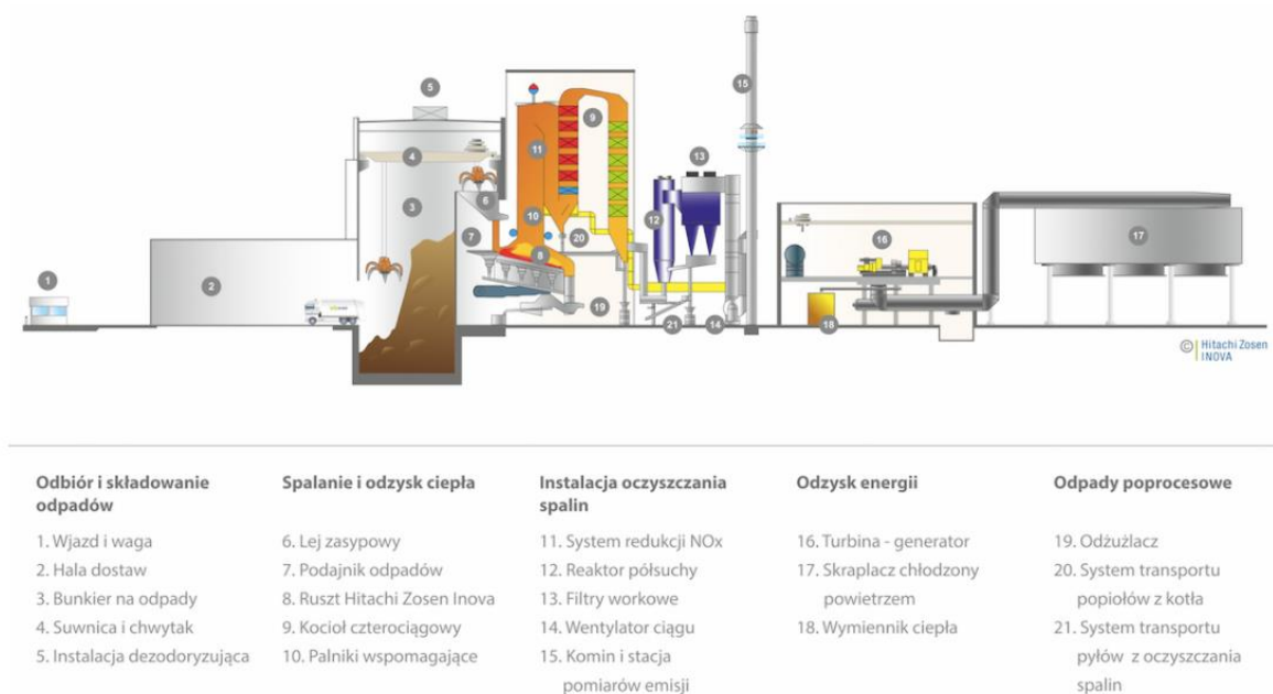
Rysunek 5. Schemat procesu przetwarzania odpadów w ITPOK
